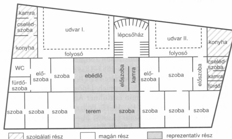
A két első emeleti lakás alaprajza a Sugárút (Andrássy út) belvárosi szakaszán az 1880-as években épült bérházban
